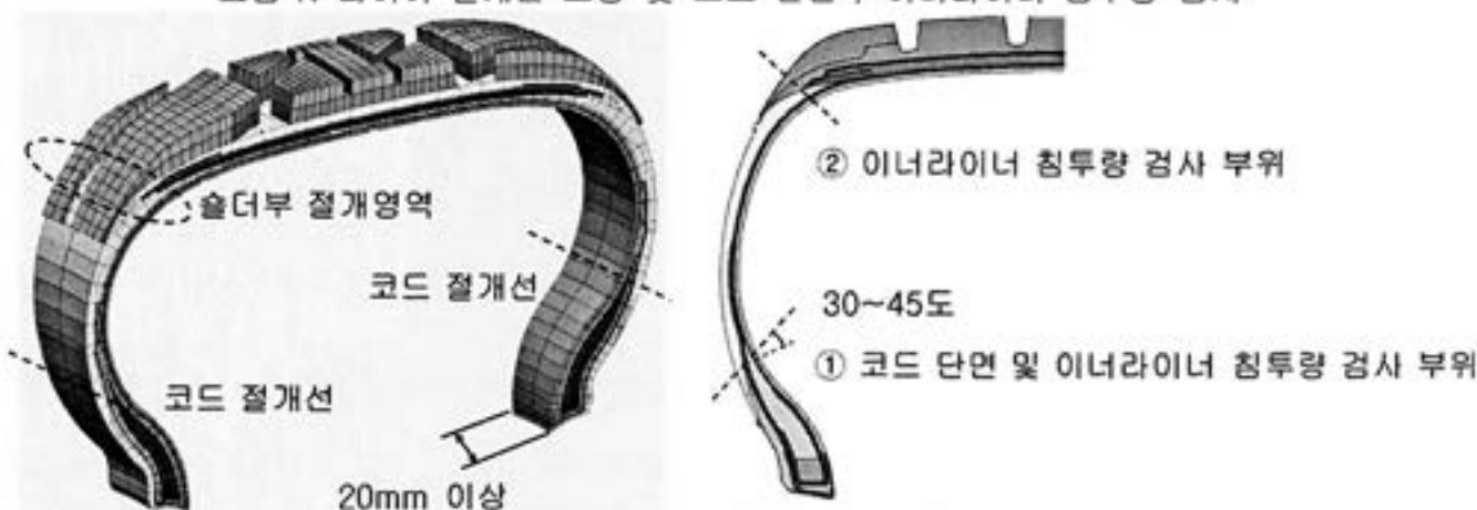
그림 1. 타이어 절개면 모형 및 코드 단면 / 인너라이너 침투량 검사
