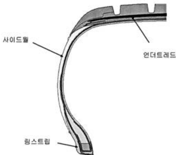
그림 2. 타이어의 언더트레드, 사이드월, 림스트립 부위
